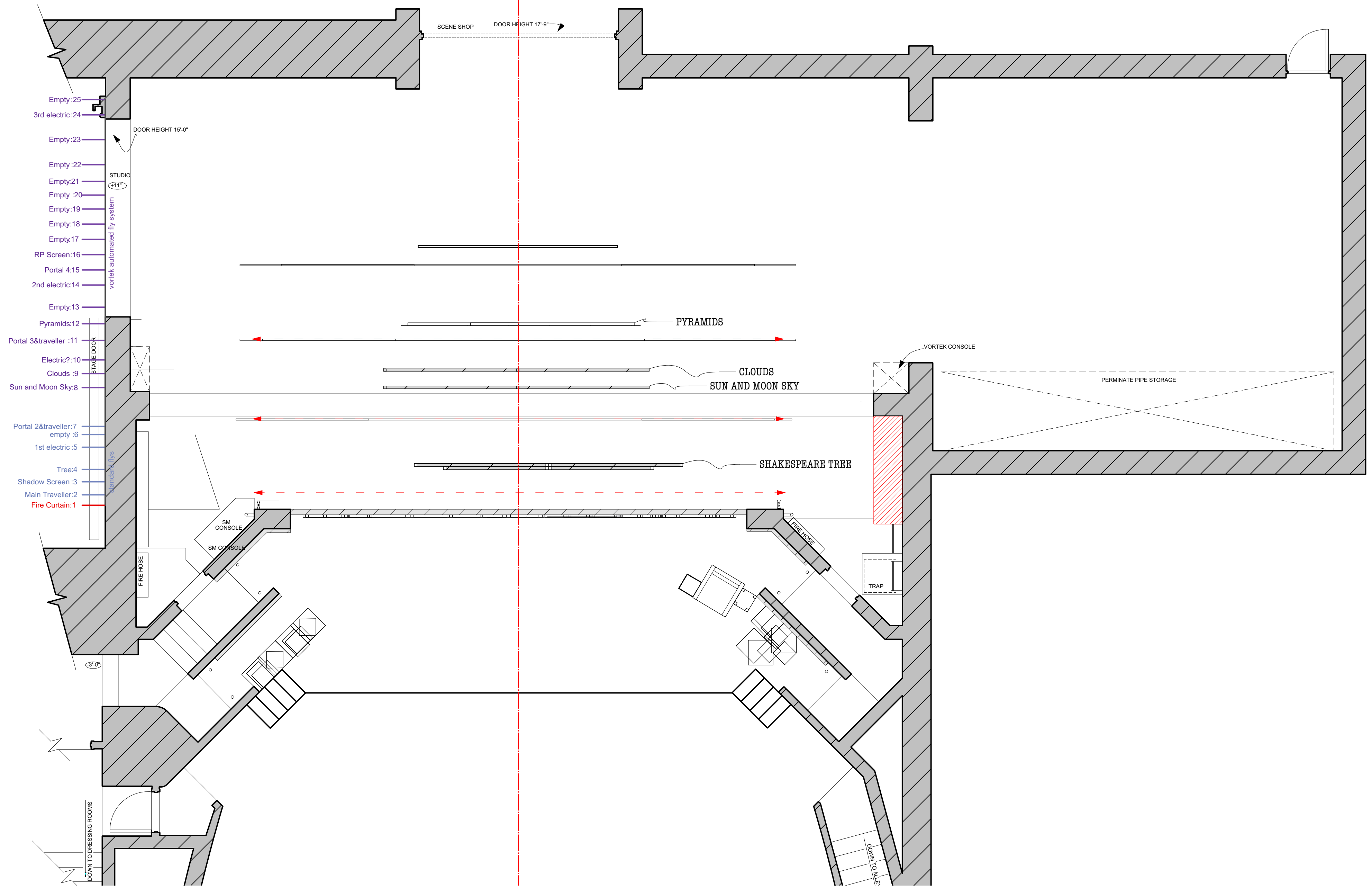
1 GROUNDPLAN Scale: 1/4" = 1'-0"
