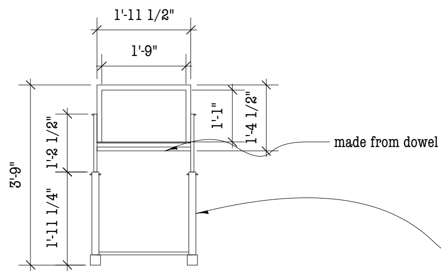
1 Front Elevation Scale: 1/2" = 1'-0"
