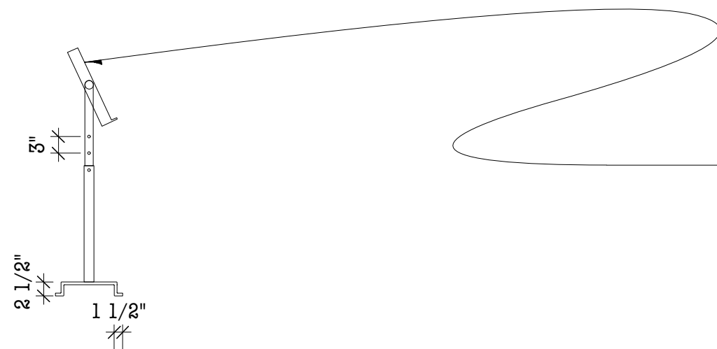
4 Side View Scale: 1/2" = 1'-0"
