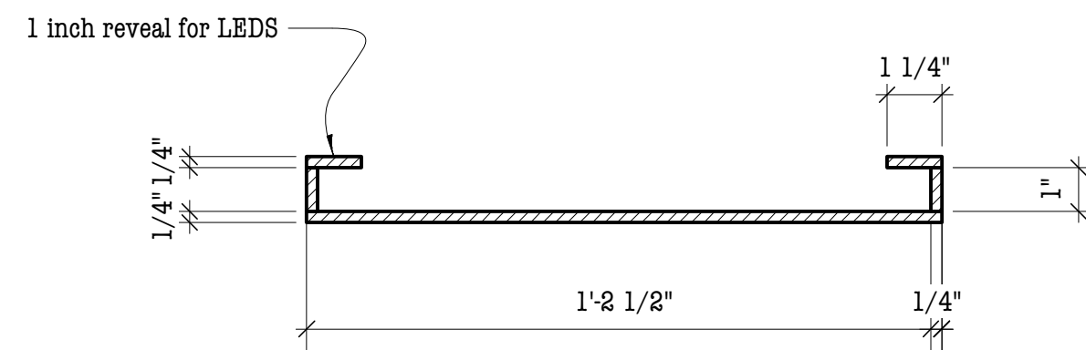
5 Box Interior Scale: 3" = 1'-0"
